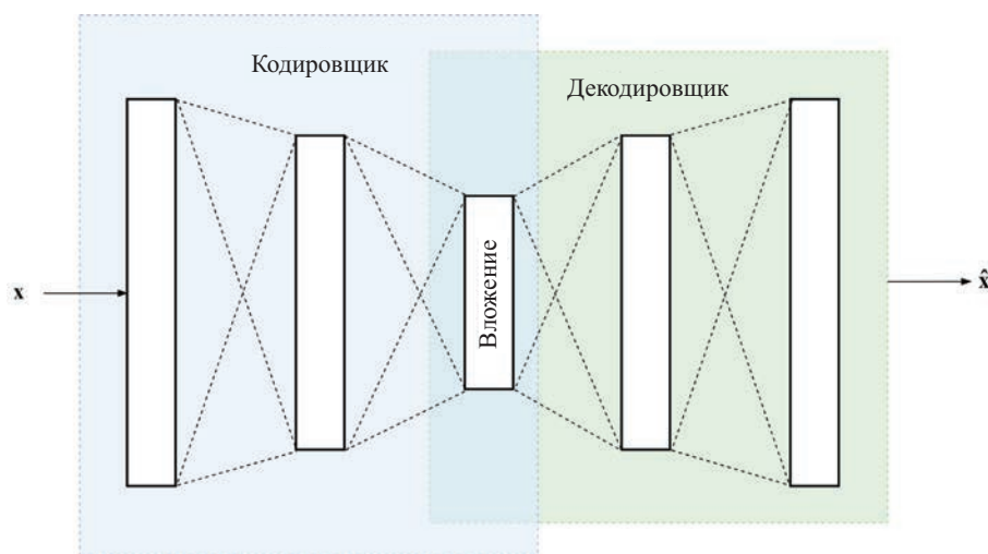
Рис. 7.6. Автокодировщик
